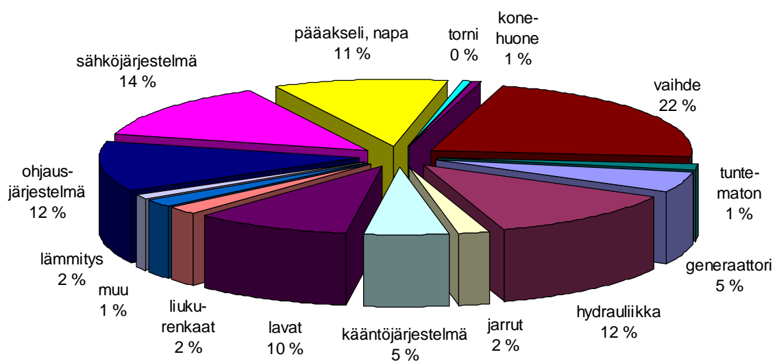
Kuva 23. Vikojen aiheuttamien käyttökätköjen jakautuminen tuulivoimaloiden eri komponenteille vuosina 1996–2010.
