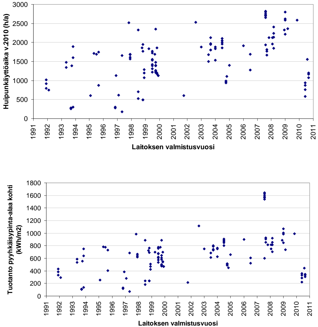
Kuva 14. Kaikkien laitosten tuotanto vuonna 2010 huipunkäyttöaikana ja suhteessa pyyhkäisy-pinta-alaan (Vuoden 2010 aloittaneet laitokset olivat vain osan vuotta toiminnassa. Tornion uudet laitokset eivät ole tässä vertailussa mukana, koska niiden tuotanto alkoi vasta vuoden viimeisinä päivinä).
